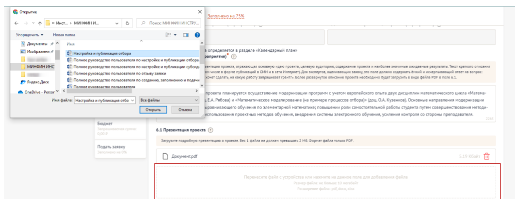
Рисунок 46. Диспетчер загрузки
