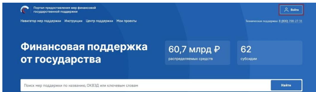
Рисунок 2. Кнопка «Войти»
