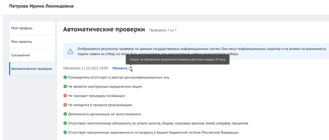
Рисунок 23. Кнопка «Обновить»
