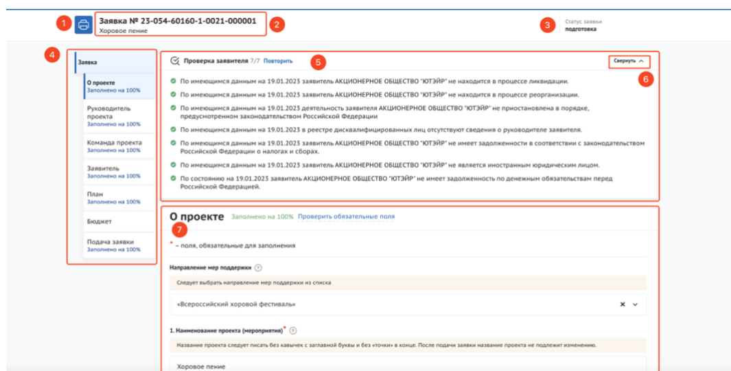
Рисунок 41. Страница заявки
