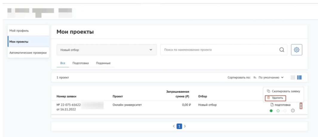
Рисунок 80. Удаление заявки
