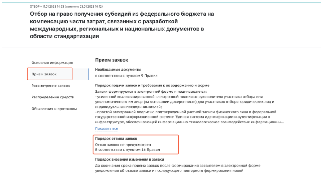
Рисунок 85. Страница отбора
