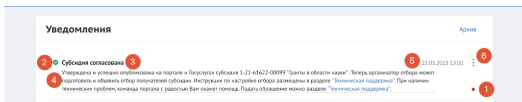
Рисунок 38. Страница «Уведомления»
