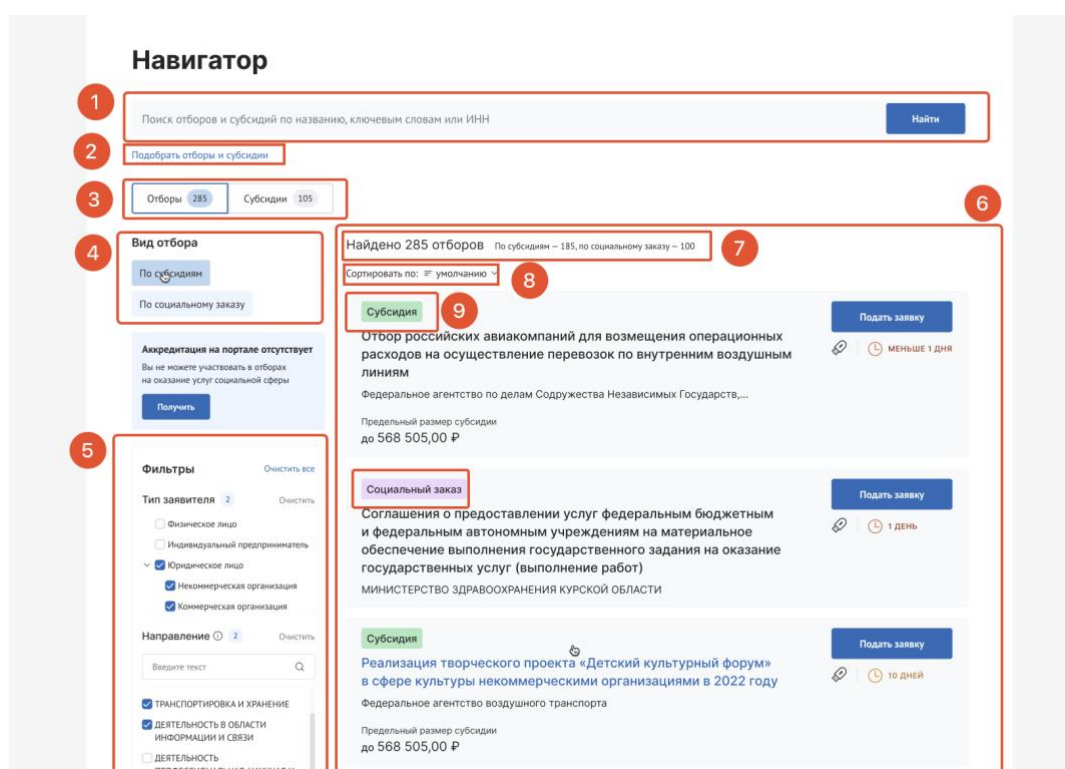
Рисунок 34. «Навигатор»
