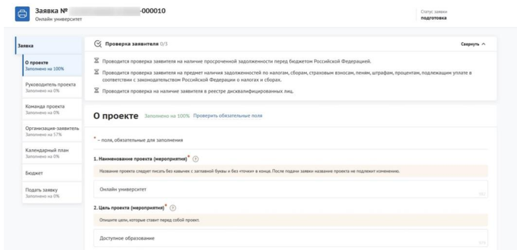
Рисунок 79. Скопированная заявка
