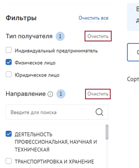
Рисунок 35. Кнопка «Очистить»
